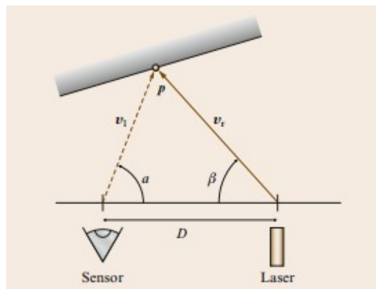
Рис 3. Схема работы триангуляционного лазерного дальномера.
